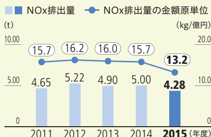
NOx排出量と原単位
