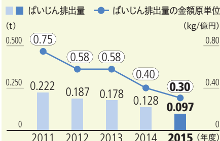
ばいじん排出量と原単位
